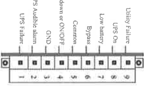
9-pin port
